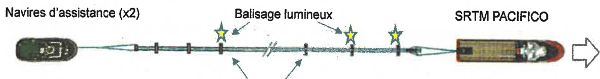
Schéma indicatif de la configuration de remorquage des sections de conduite (270m et 700m)
