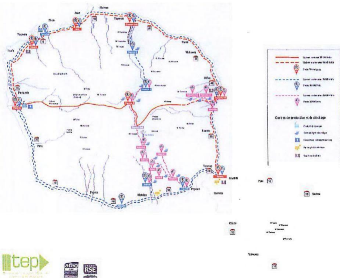
Figure 15 : Le réseau de transport électrique à Tahiti en 2030
