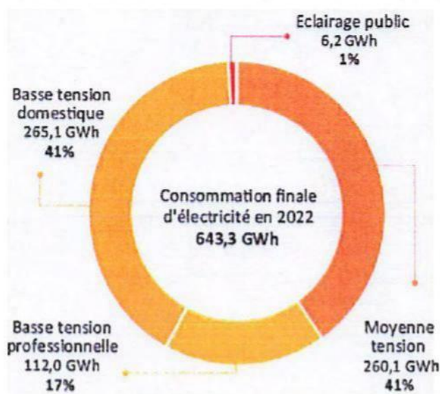
Figure 12 : Typologie des consommateurs d'électricité en 2022 - Sources : OPE, EDT 2022
